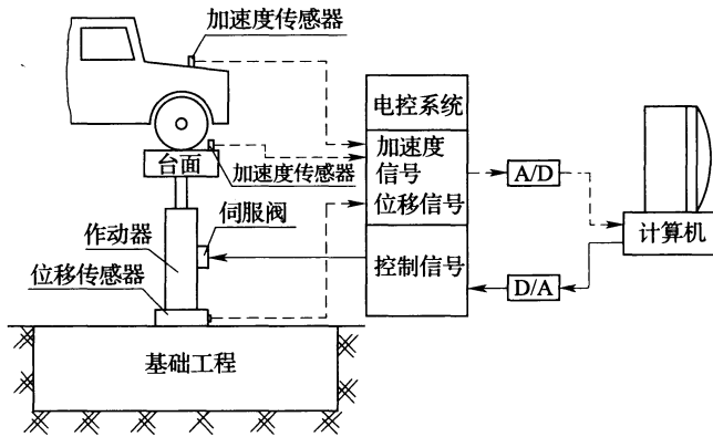
图 3 电液伺服振动台原理框图
