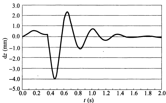
图 1 锻锤隔振基础动力响应
