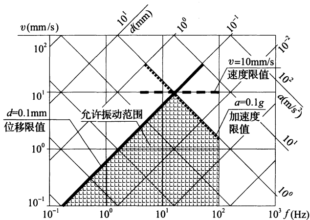
图 4 电液伺服试验台基础容许振动幅值
