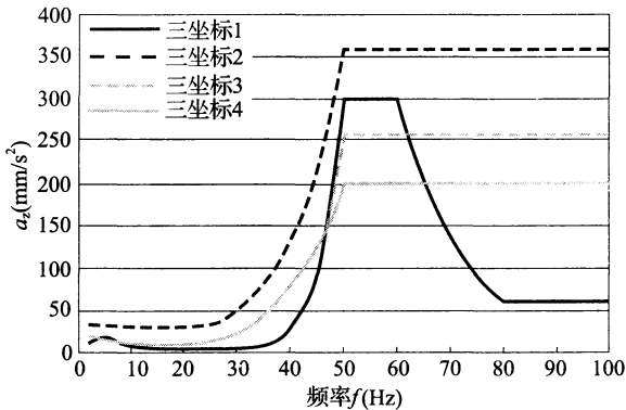
图 2 三坐标测量机的容许振动值
